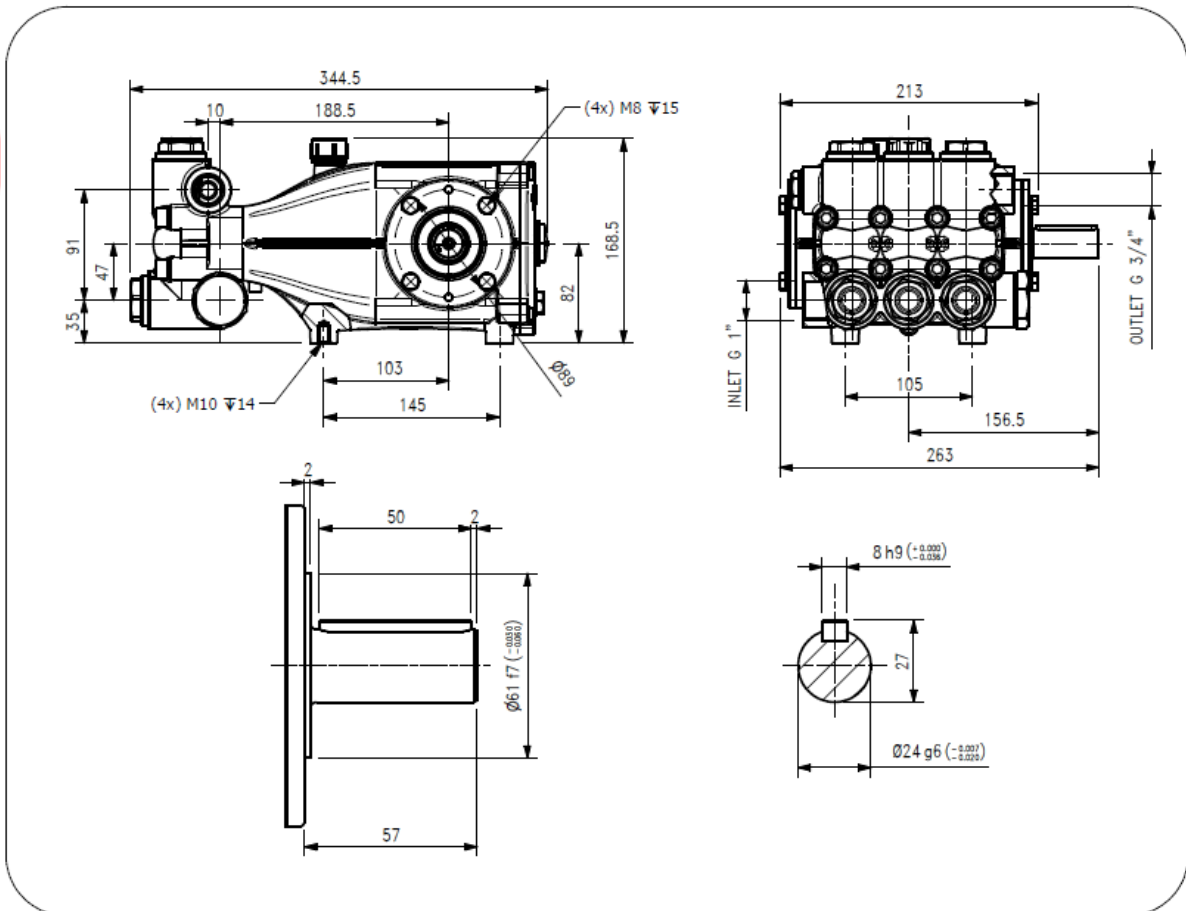
Dimensioni d'ingombro
